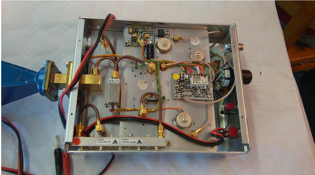
Hjemmebygget 10 GHz udstyr
