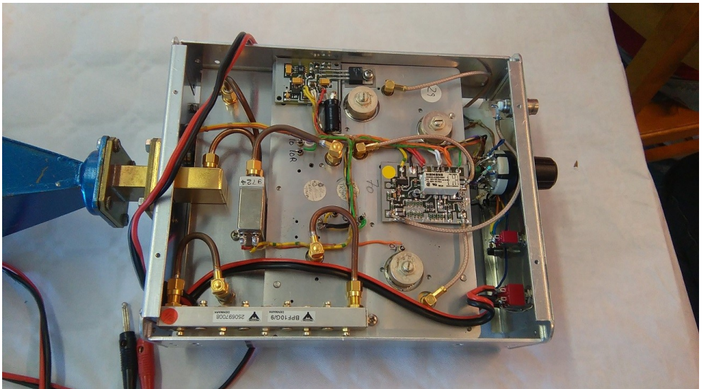
Hjemmebygget 10 GHz udstyr, OZ2OE
